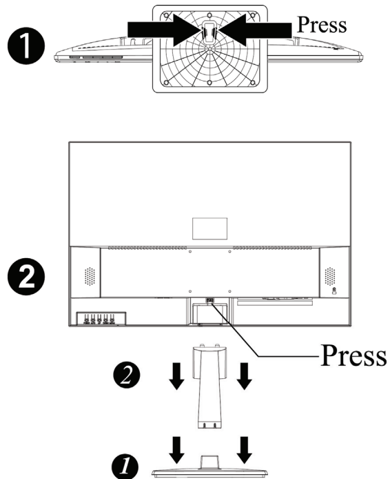
ABBILDUNG 1. INSTALLIEREN UND ENTFERNEN DES STÄNDERS
