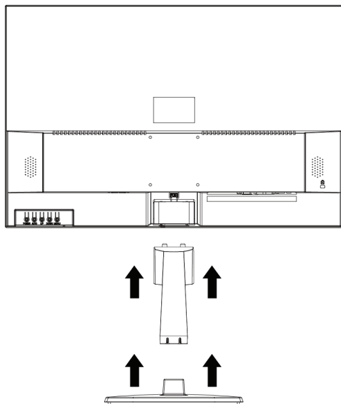
ABBILDUNG 1. INSTALLIEREN UND ENTFERNEN DES STÄNDERS
